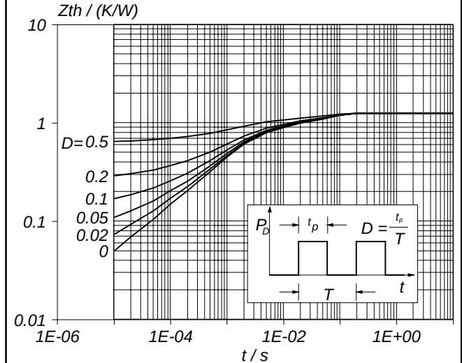
Fig.11. Transient thermal impedance. Z_{th\ j-hs} = f(t) ; parameter D = t_p/T
